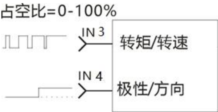
图 4.6.1 100%占空比+方向控制
